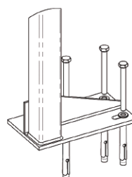
DETALLE C Fijación Bastidor a suelo
