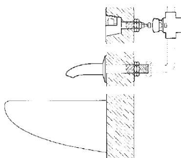
PRESTO 127 TC PULSADOR 18400 CAÑO ANTIRROBO 30800
