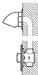
PRESTO 555 TC ROCIADOR ANTIVANDÁLICO (instalación empotrada)
