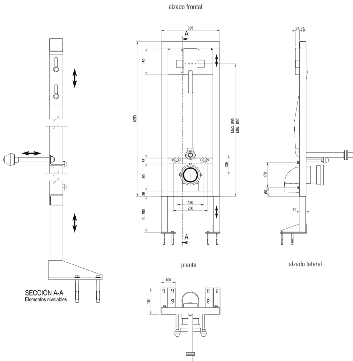
DETALLES DE INSTALACIÓN
