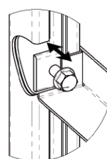
DETALLE A Nivelación elementos
