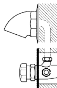
PRESTO MEZCLADOR ALPA ROCIADOR ANTIVANDÁLICO (instalación empotrada)
