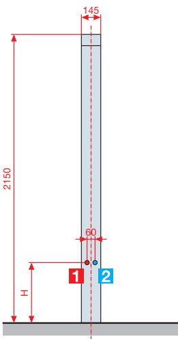
Ducha fija / Chuveiro fixo 250x250 mm
