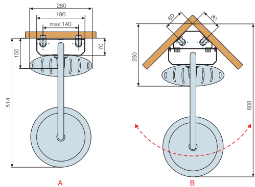
Ducha fija / Chuveiro fixo 200x200 mm
