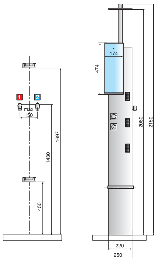
Ducha fija / Chuveiro fixo 250x250 mm
