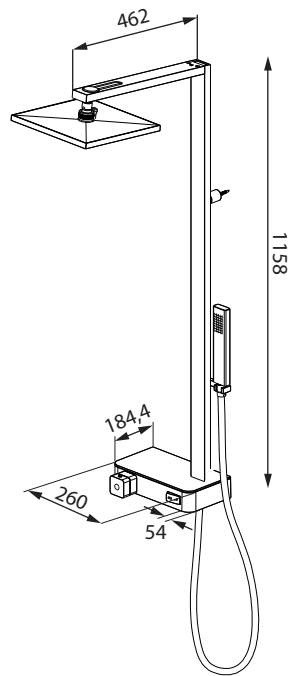
Ducha fija / Chuveiro fixo 250 x 250 mm
