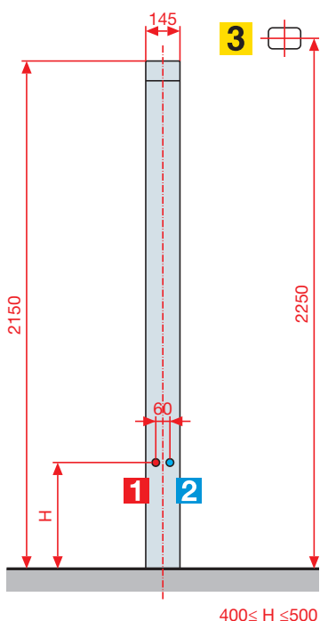
Ducha fija / Chuveiro fixo Ø 120 mm
