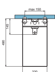
Versión a pared Montagem à parede
