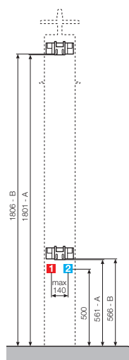
Ducha fija / Chuveiro fixo 200x200 mm
