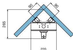
Versión en ángulo Montagem de angulo
