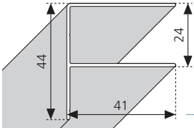
ROSE ROSSE H 200 cm
