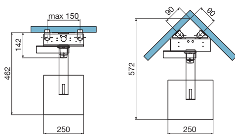
Ducha fija / Chuveiro fixo 250x250 mm
