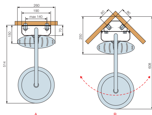
Ducha fija / Chuveiro fixo 200x200 mm
