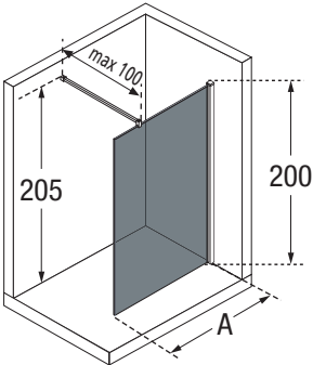
Pieza de sujeción del cristal a suelo Peça de fixação do vidro ao chão
