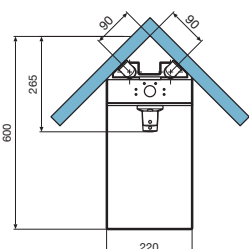
Versión en ángulo Montagem de angulo
