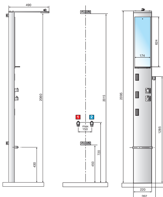
Ducha fija / Chuveiro fixo 220x145 mm
