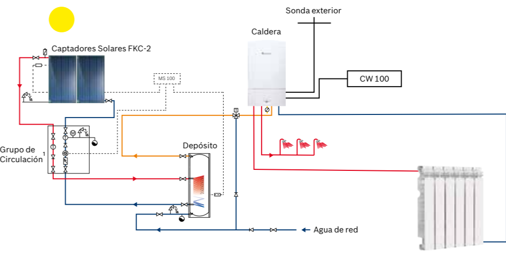
Instalación de a.c.s. y calefacción central con sistema de circulación forzada con depósito de un serpentín y apoyo de caldera.
