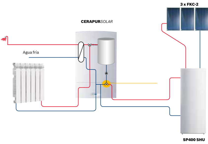
Instalación de a.c.s. y apoyo solar para calefacción con Cerapur Solar y depósito SP 400 SHU.
