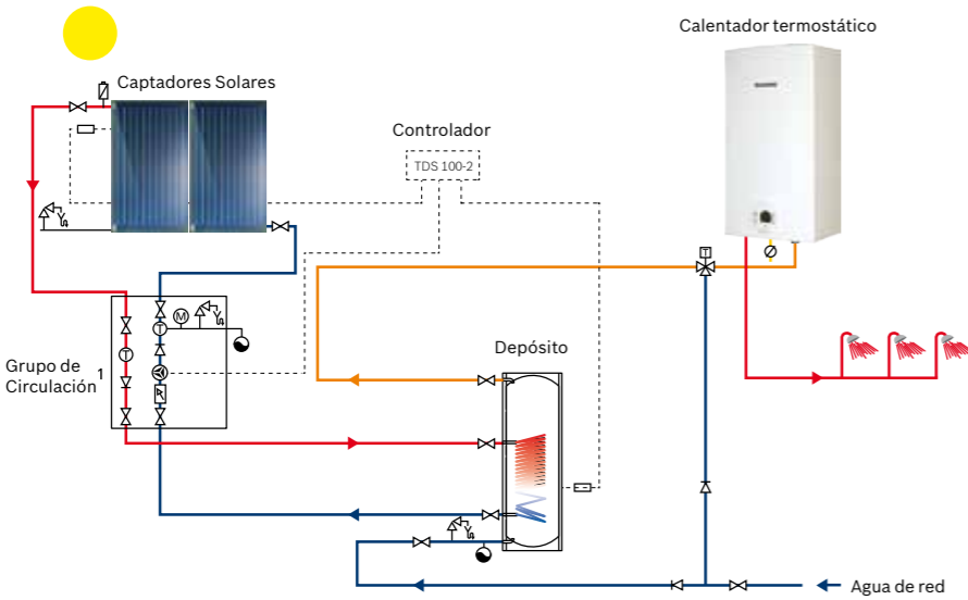
Instalación de a.c.s. a través de sistema de circulación forzada con depósito de un serpentín y apoyo de calentador.
