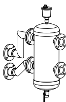
Kit botella de equilibrio para caudal máximo de 18 m³/h (conexión DN 65)
