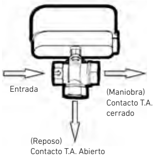
Válvula de zona motorizada de 3 y 2 vías
