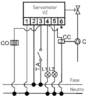
Conexiones eléctricas
