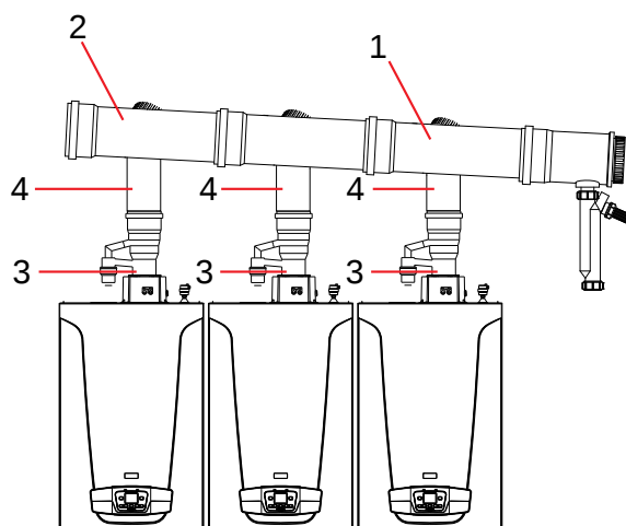
Kit evacuación cascada gamas Bios Plus/Power HT Plus
