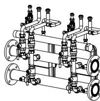
Kit hidráulico doble (para 2 calderas)
