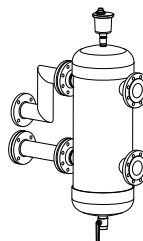
Kit botella de equilibrio para caudal máximo de 28 m³/h (conexión DN 80)
