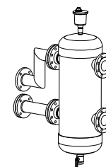
Kit botella de equilibrio para caudal máximo de 28 m³/h (conexión DN 80)
