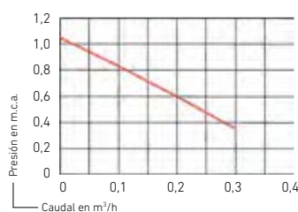
Curva característica
